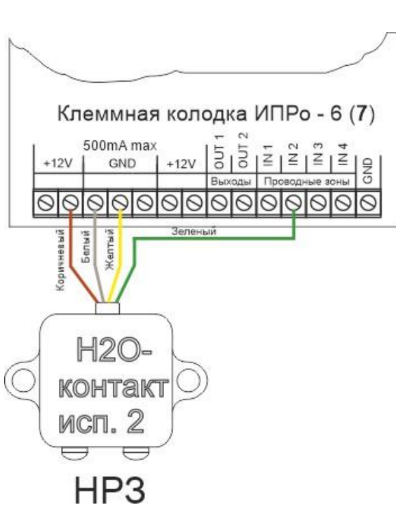
Подключение 1 датчика
