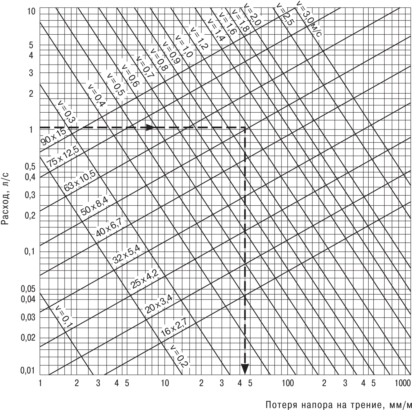
Номограмма 2 для определения потерь напора в трубах SDR6, SDR5
