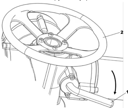
Рис. 5. Переключение на ручное управление.
