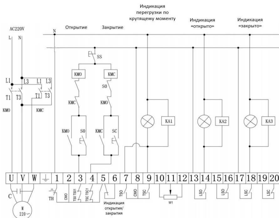
Электрическая схема 220В.
