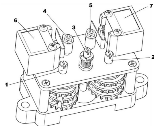
Рис. 4. Механизм концевых выключателей.
