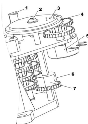
Рис. 6. Механизм положения
