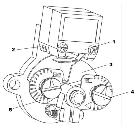
Рис.3. Механизм управления крутящим моментом
