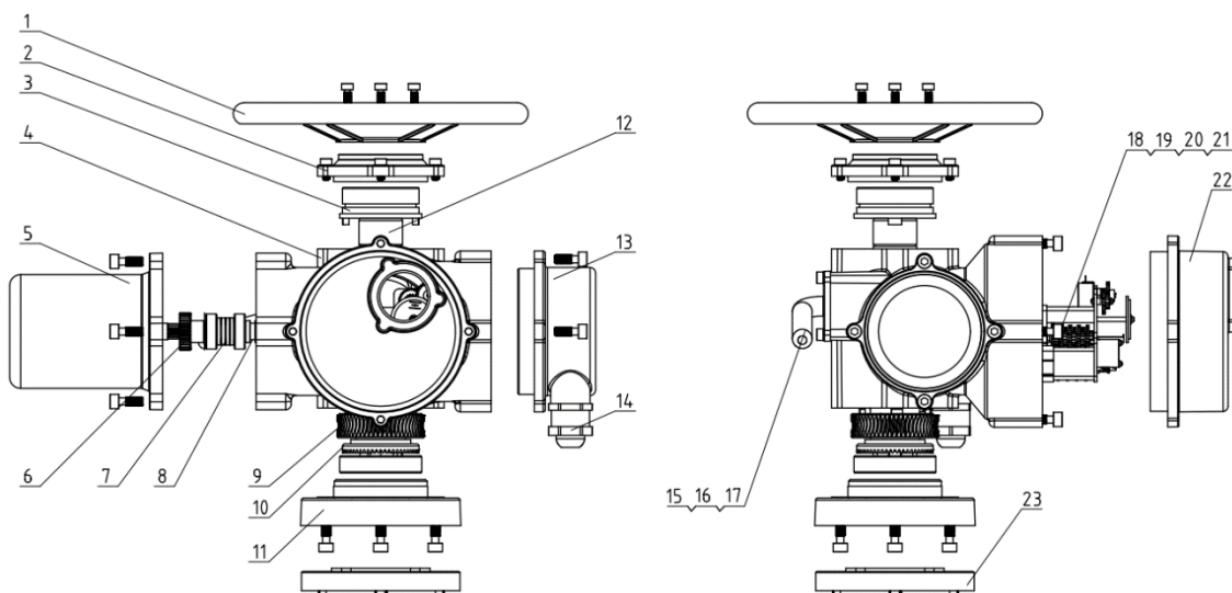
Рис. 2. Внутреннее устройство электропривода S-70 – S-1200
