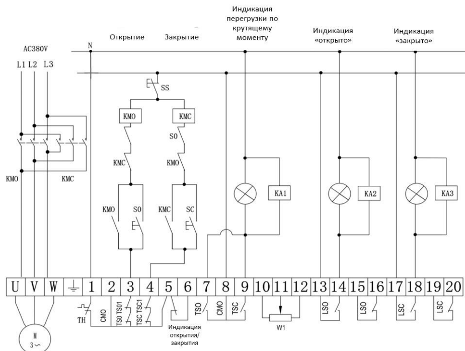
Электрическая схема 380В.
