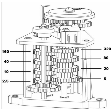
Рис.7. Настраиваемое количество оборотов на механизме положения.
