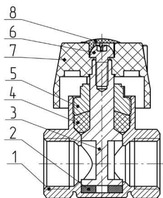
Рисунок 2 – Конструкция крана
