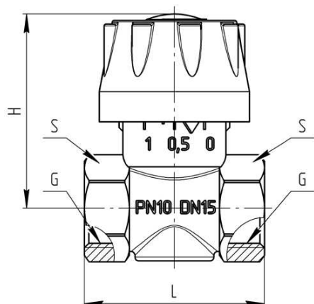
Рисунок 3 – Габаритные размеры крана.
