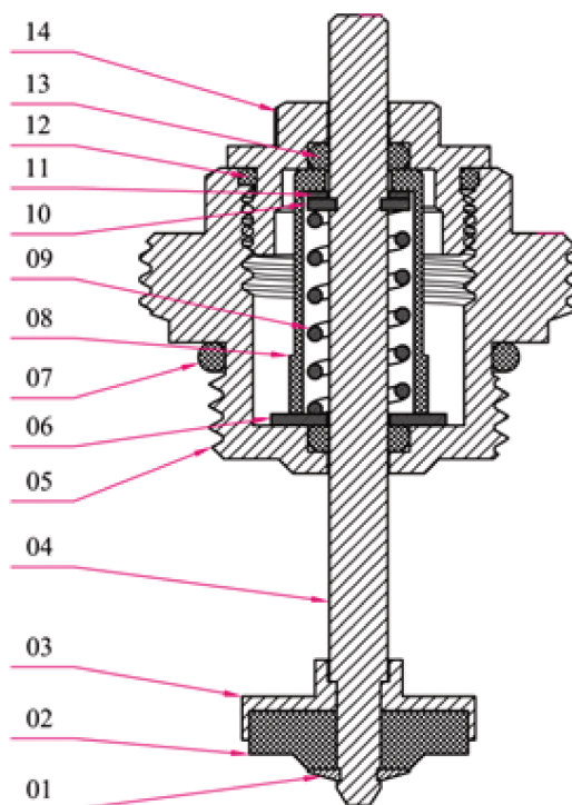
Рисунок 3. Конструкция регулировочного клапана коллектора 9501
