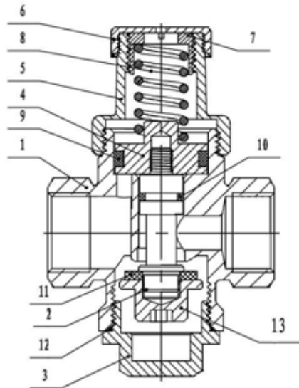
Рис 1. Основные элементы конструкции
